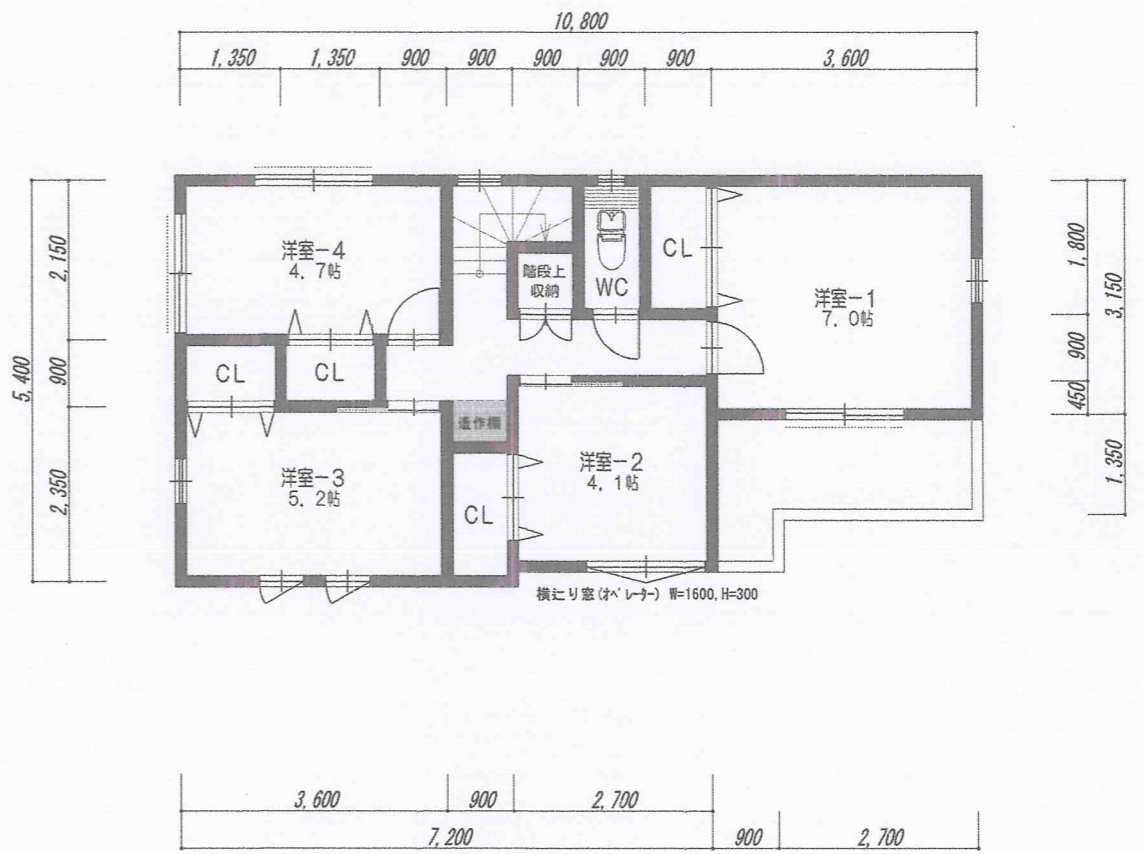
2階平面図 1/100
