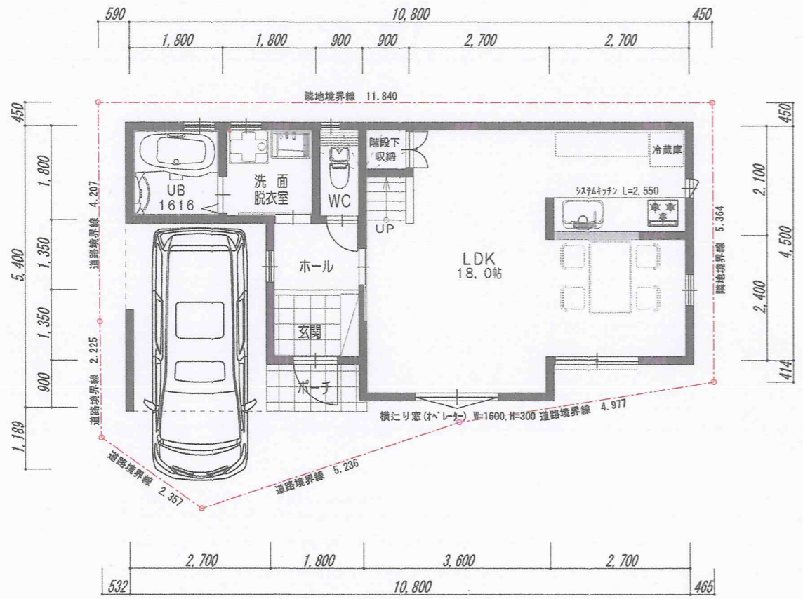
1階平面図 1/100
